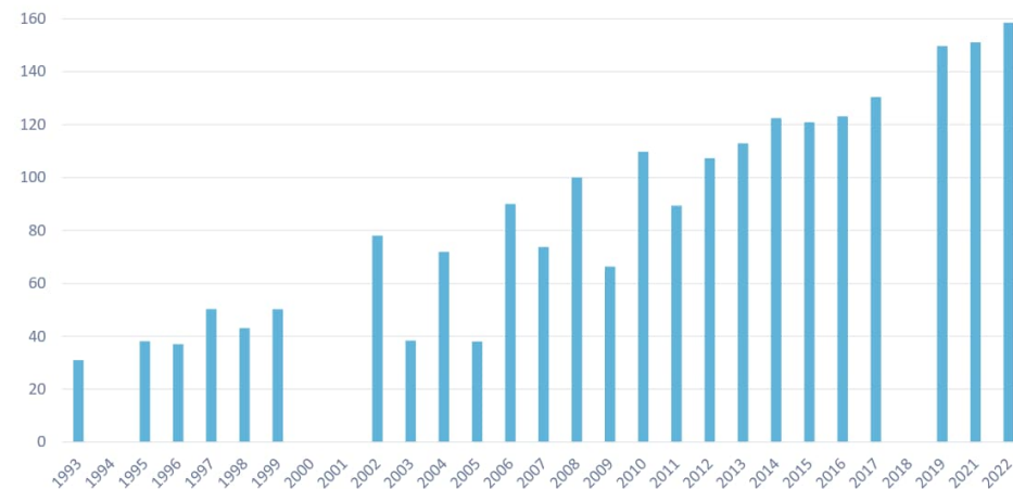
Asennettujen voimaloiden roottorin keskimääräinen halkaisija (m)
